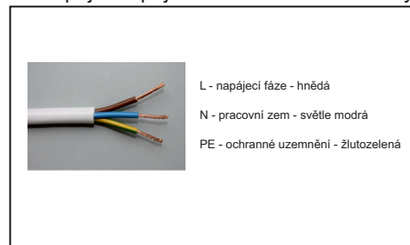
6. Připojte napájecí kabel varianta třížilový.
