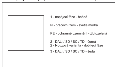
7. Připojte napájecí kabel varianta pětižilový.
