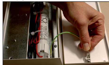
3. Odpojte zemní vodič.
